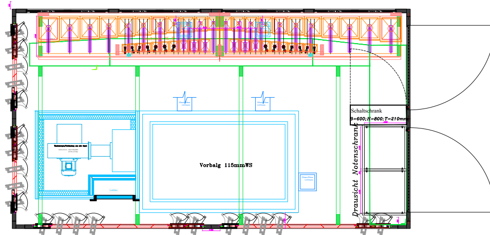
Draufsicht - Windanlage
